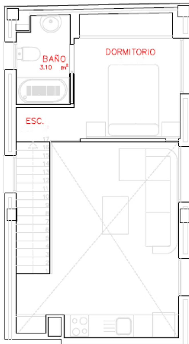
PLANTA ALTA
