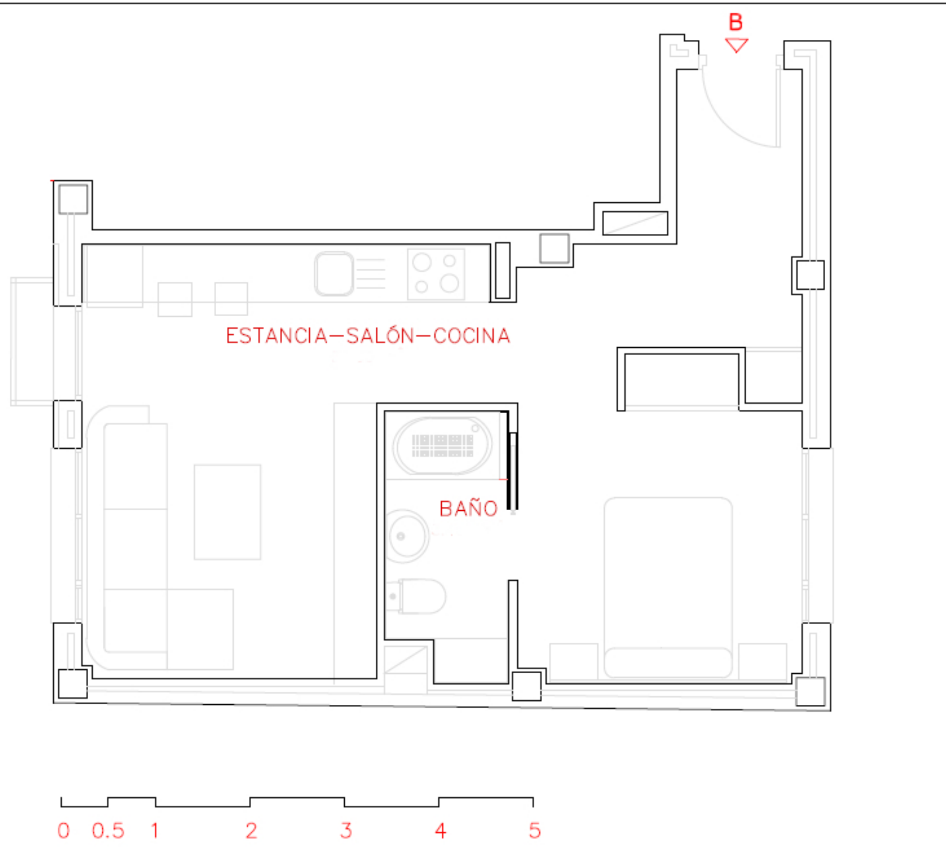
VIVIENDA B, PLANTA 2ª
